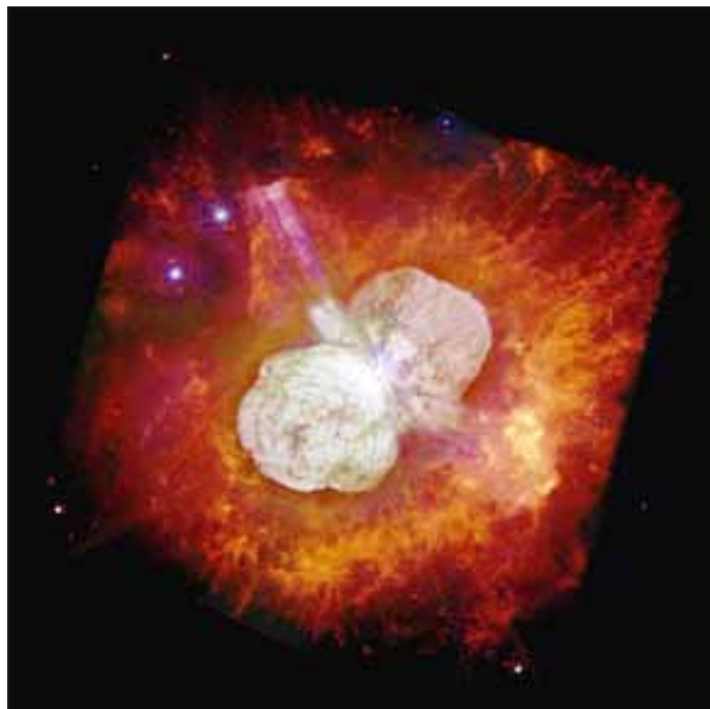
Eta Carinae, una de las estrellas más masivas de la galaxia que se encuentra dentro de la Nebulosa de Carina y que da el nombre a este proyecto, captada por el telescopio espacial Hubble.
